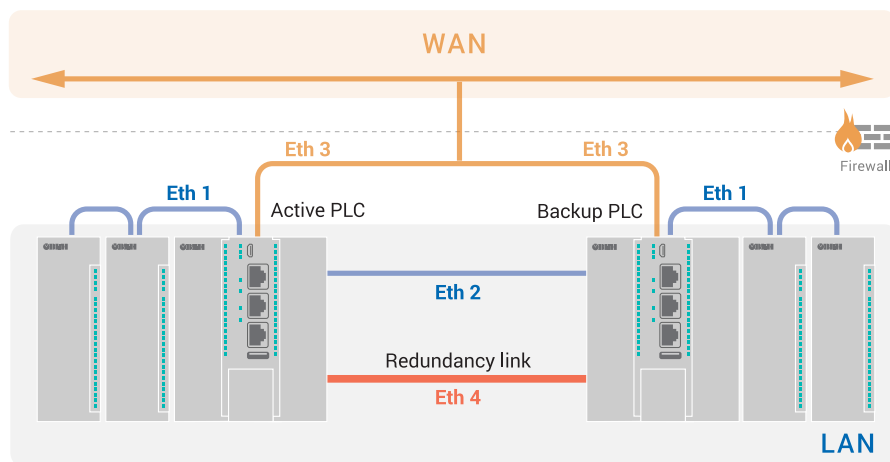
Рис. 2-17: Схема №5 сетевых портов контроллера ПЛК210 с поддержкой функции резервирования
