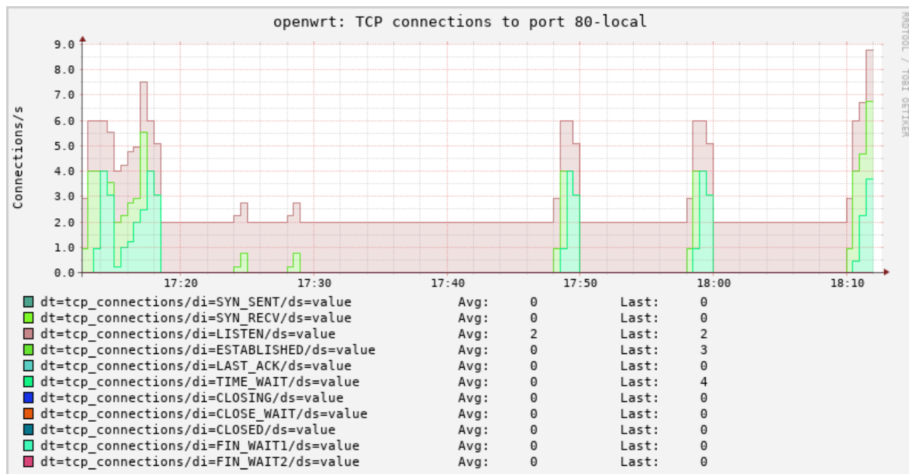
Рис. 8-18: Статистика. График открытых соединений для TCP порта
