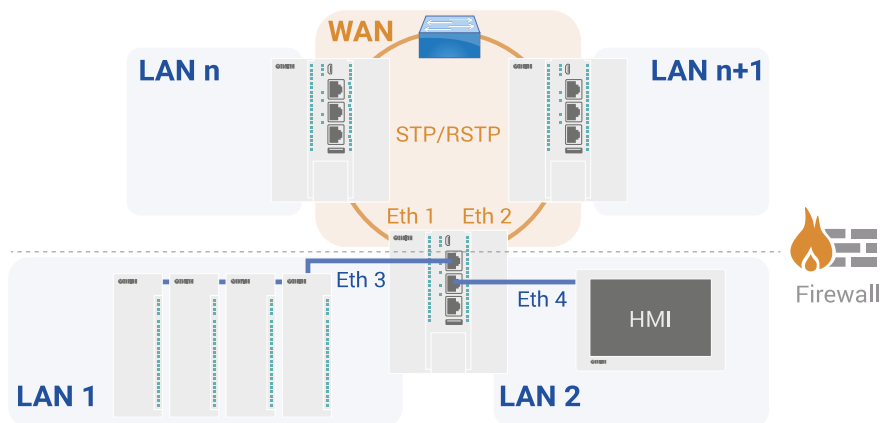
Рис. 2-13: Схема №2 сетевых портов контроллера ПЛК210
