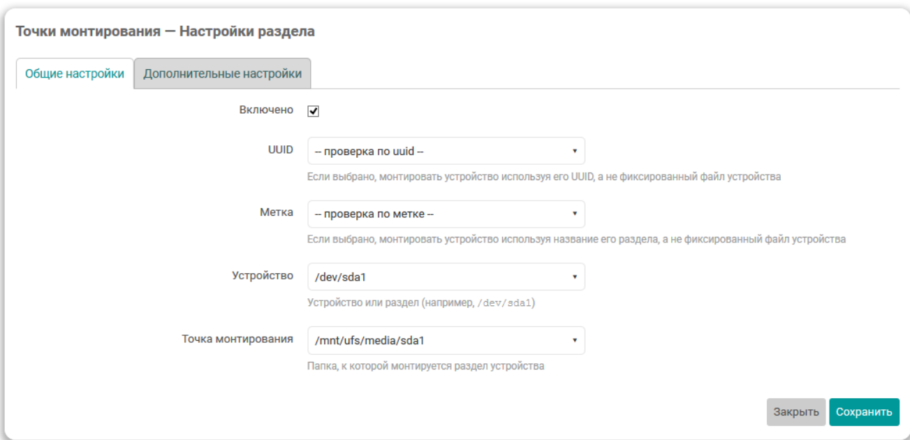
Рис. 4-15: Общие настройки точки монтирования раздела
