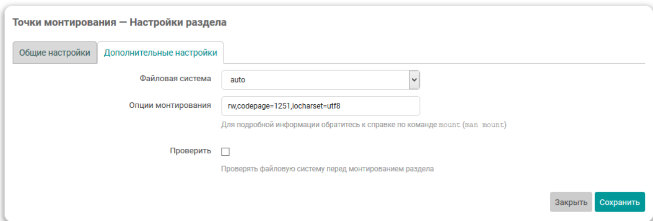
Рис. 4-16: Дополнительные настройки точки монтирования раздела
