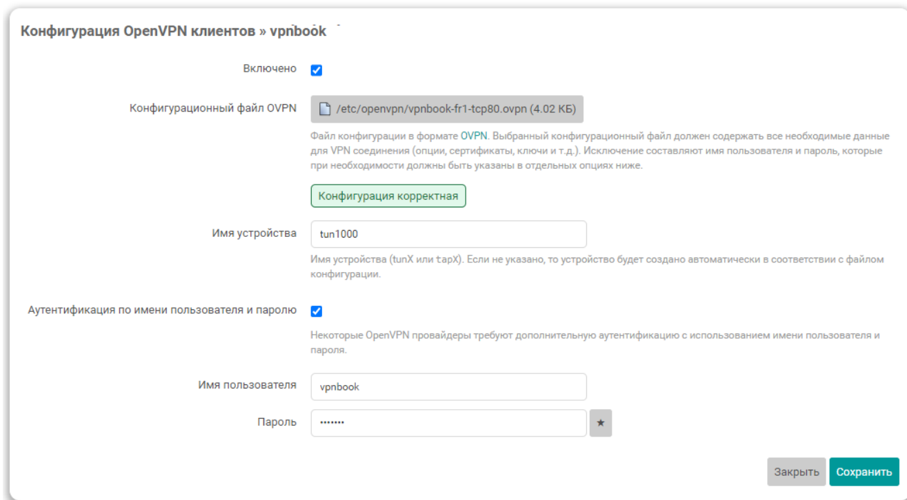
Рис. 6-36: Всплывающее окно редактирования настроек экземпляра OpenVPN клиента
