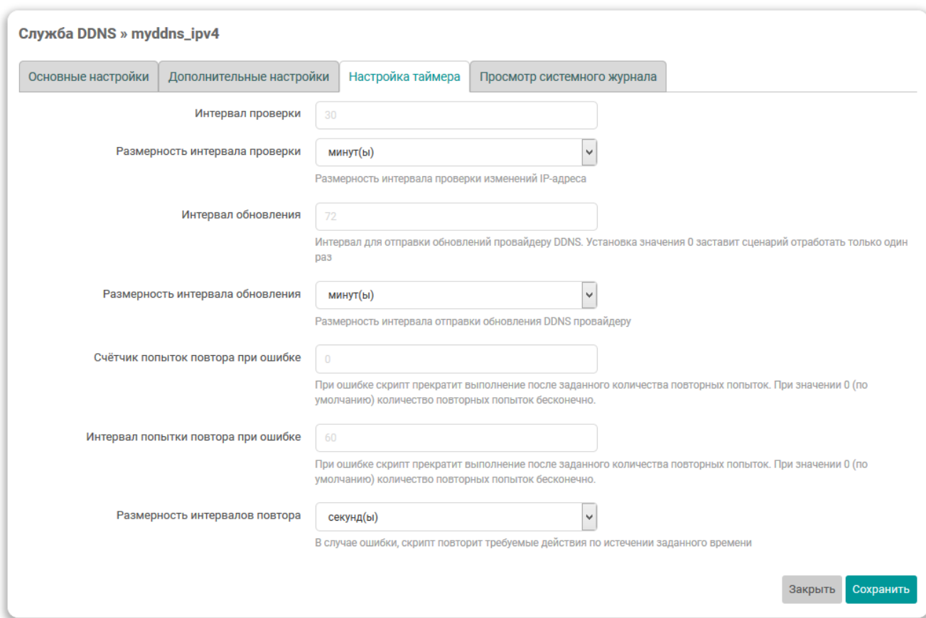
Рис. 6-13: Вкладка «Настройки таймера» окна редактирования DDNS службы
