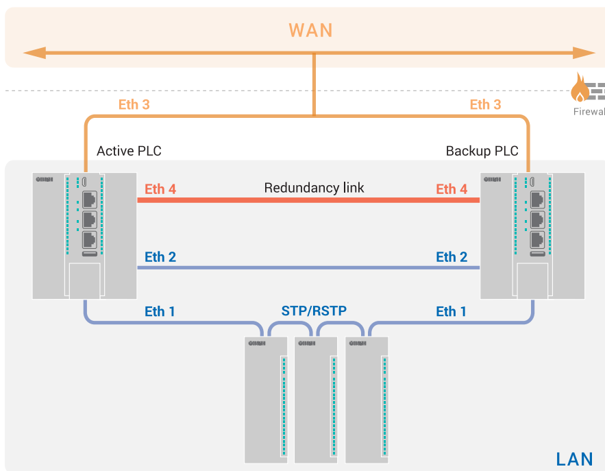
Рис. 2-16: Схема №4 сетевых портов контроллера ПЛК210 с поддержкой функции резервирования
