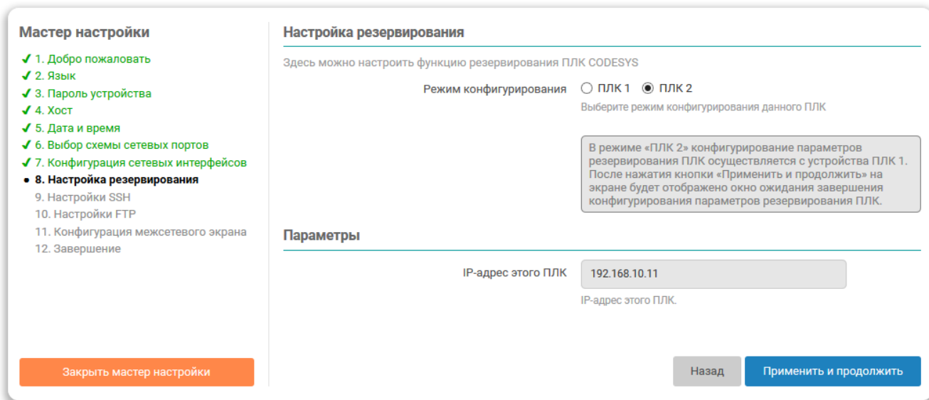
Рис. 2-28: Мастер настройки. Настройки резервирования в режиме конфигурирования «ПЛК 2»
