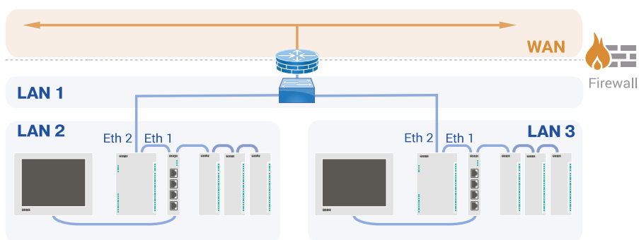
Рис. 2-10: Схема №3 сетевых портов контроллера ПЛК200
