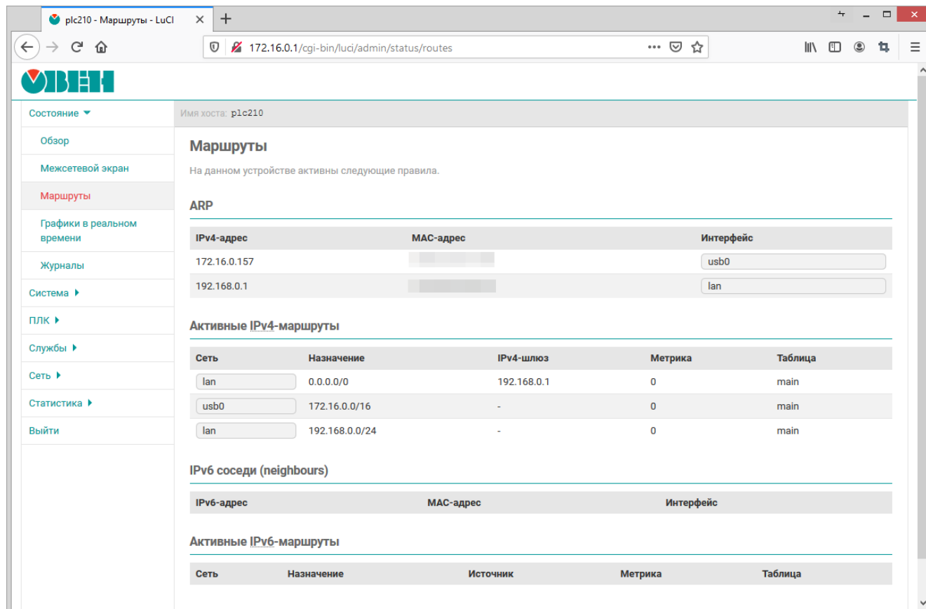
Рис. 3-14: Страница «Маршруты»
