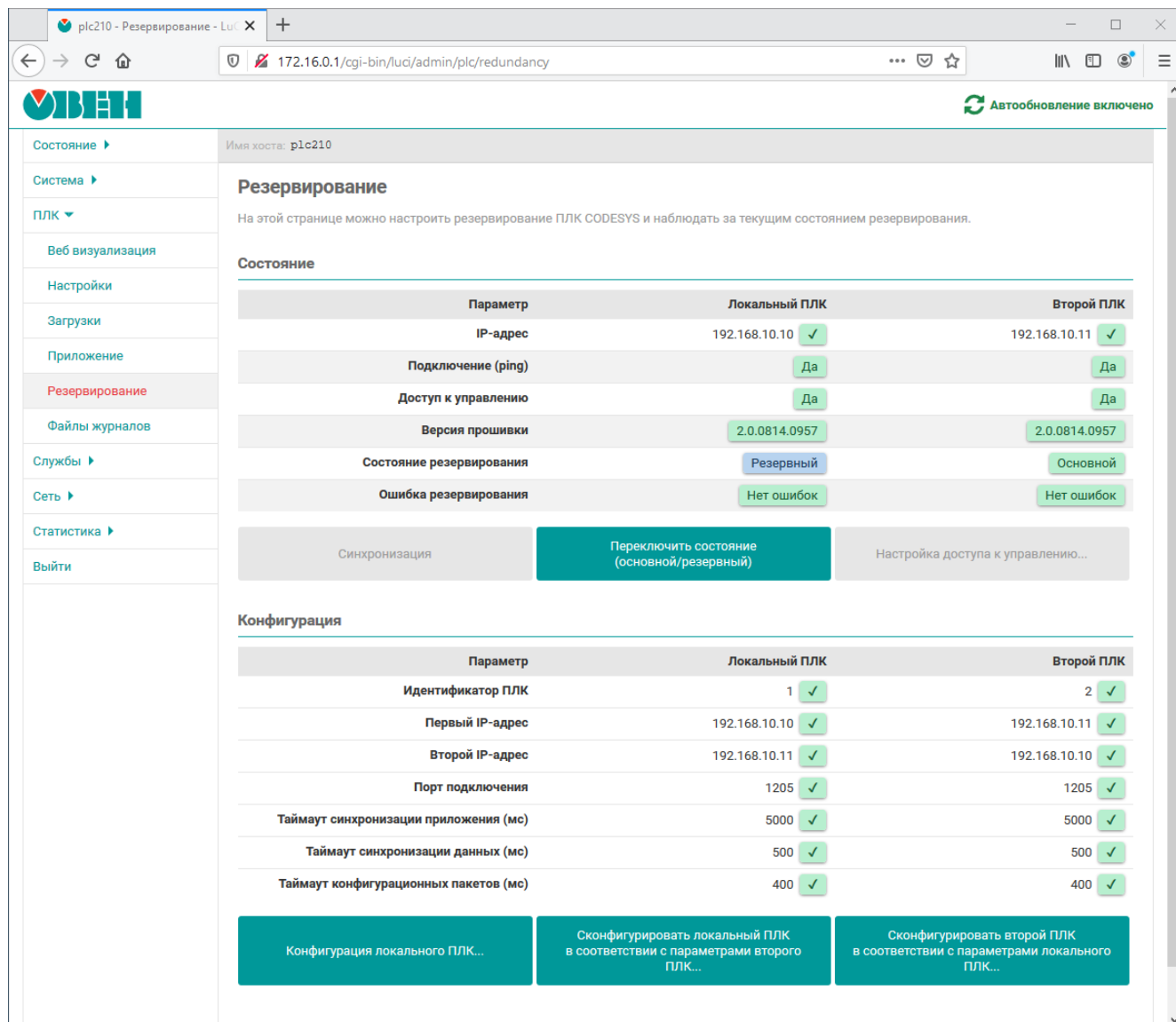
Рис. 5-27: Страница «Резервирование»
