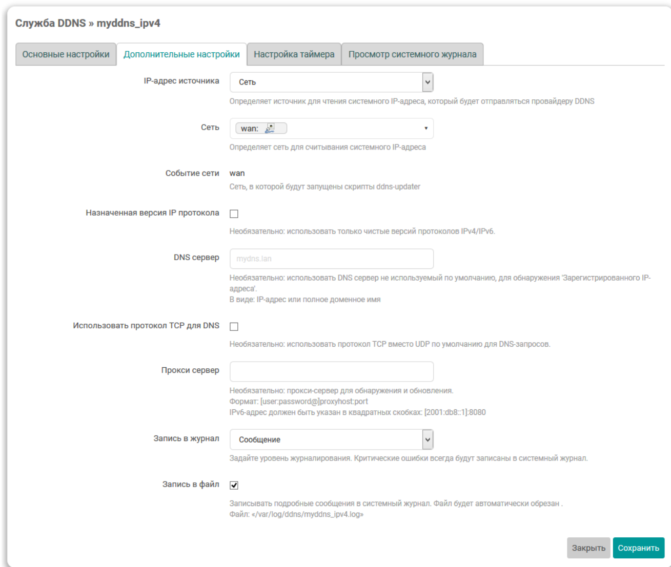
Рис. 6-8: Вкладка «Дополнительные настройки» окна редактирования DDNS службы
