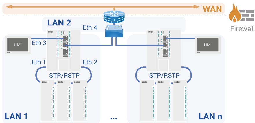
Рис. 2-14: Схема №3 сетевых портов контроллера ПЛК210
