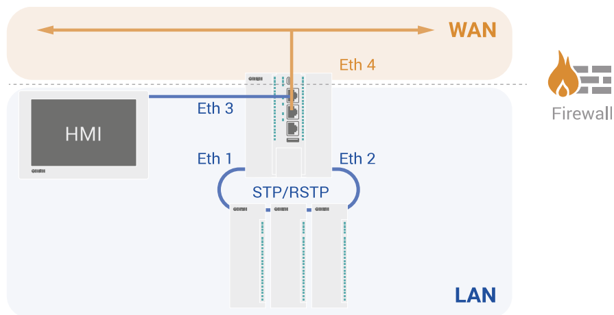
Рис. 2-12: Схема №1 сетевых портов контроллера ПЛК210
