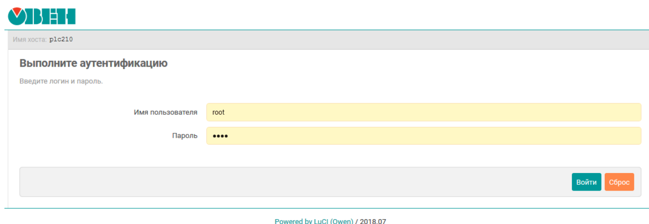
Рис. 1-2: Страница аутентификации
