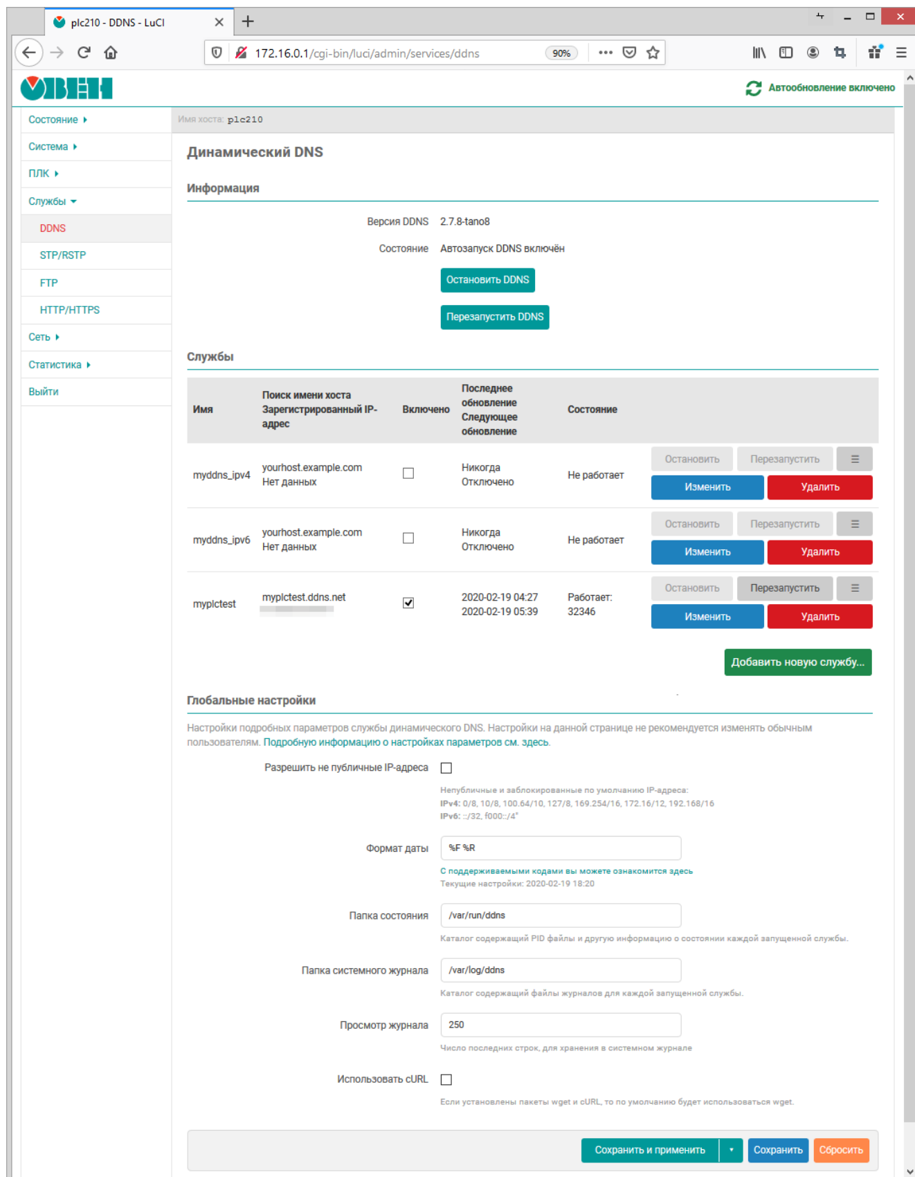
Рис. 6-3: Страница «DDNS»
